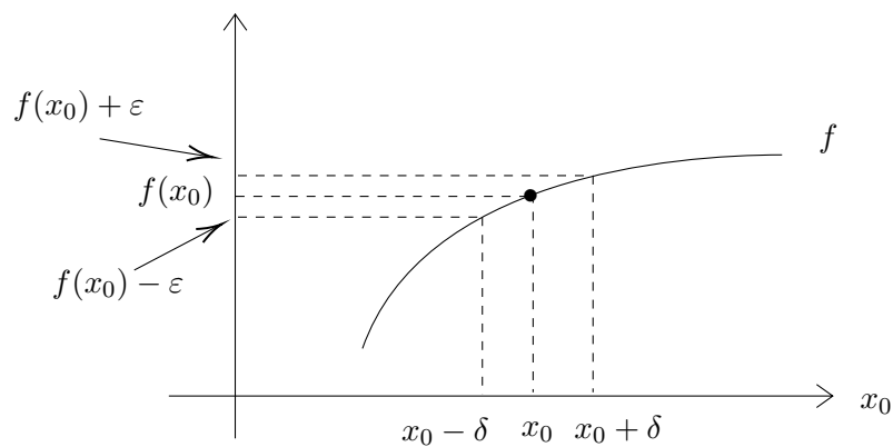
Abb. 5.13: Veranschaulichung der Stetigkeitsdefinition
