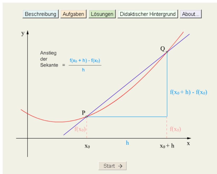
Abb. 5.7: Tangente als Grenzwert von Sekanten - interaktiv; Quelle: https://mathe-online.at/galerie/diff1/ablgrenz/index.html
