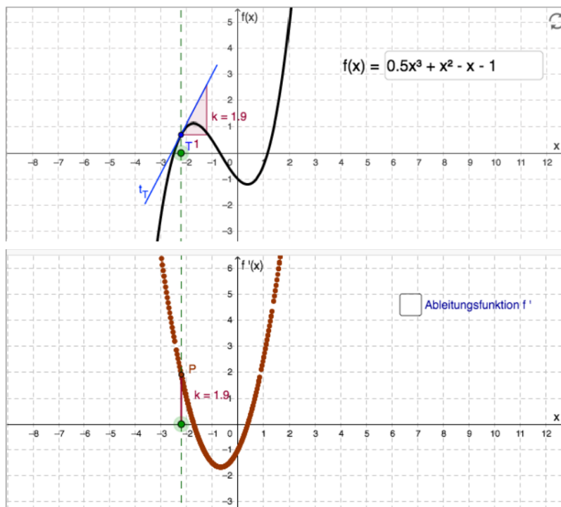
Abb. 5.36: Von der Ableitung an einer Stelle zur Ableitungsfunktion
