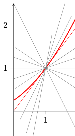
Abb. 5.23: Die Tangente als Bestapproximierende im „Geradenbüschel“ durch (x_0, f(x_0))
