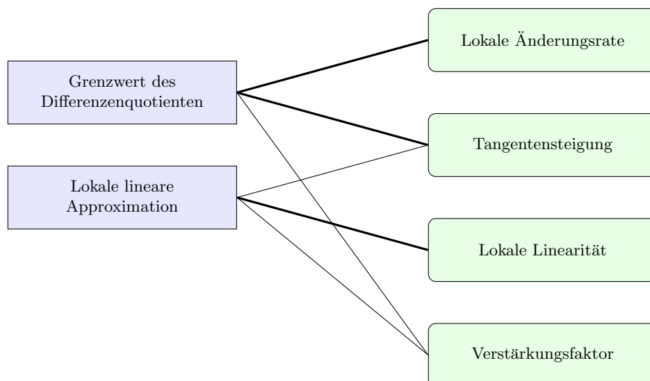
Abb. 5.34: Aspekte und Grundvorstellungen zum Ableitungsbegriff und ihre wechselseitigen Beziehungen
