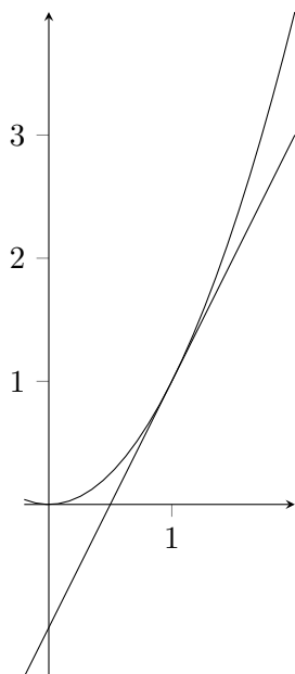
Abb. 5.22: Die Normalparabel und ihre Tangente bei P = (1, 1)
