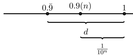
Abb. 4.38: Abstand \frac{1}{10^n} zwischen 0.9(n) und 1 für „grosses“ n .
