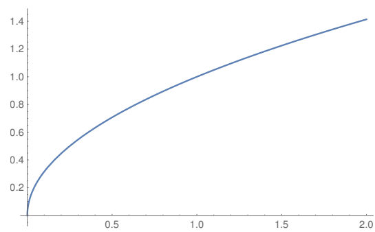
Abb. 5.19: Graph der Betragsfunktion |x| Abb. 5.20: Graph der Wurzelfunktion \sqrt{x}
