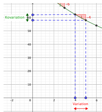
Abb. 3.7: Kovariationsvorstellung am Graphen
