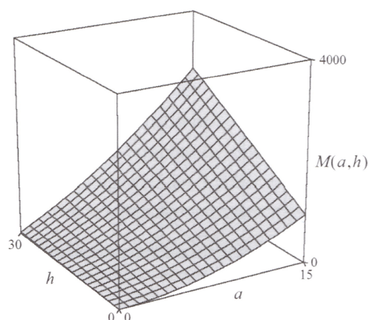
Graph von M(a, h)
