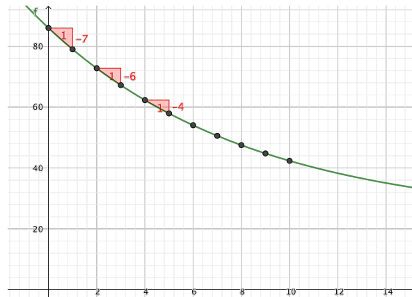
Abb. 3.5: Graphische Darstellung — Abkühlvorgang von Tee
