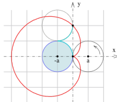
Abb. 3.14: Die Kardioide
