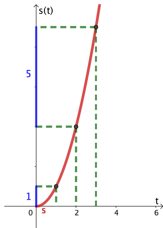
Abb. 5.10: In gleichen Zeiteinheiten zurückgelegter Weg
