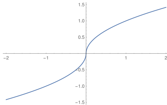
Abb. 5.21: Graph der Funktion f aus (5.29)
