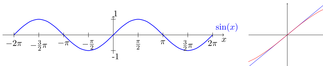
Abb. 5.25: Der Graph des Sinus und sein Verhalten bei 0
