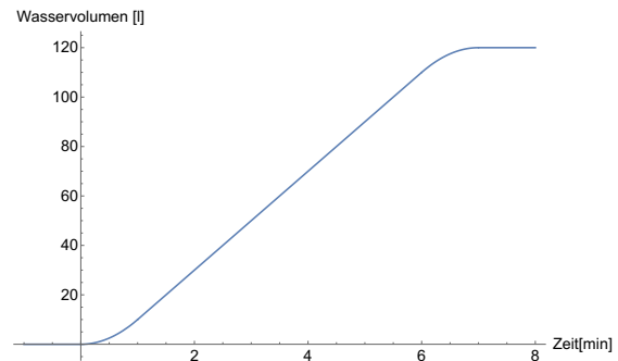
Abb. 6.5: Wasservolumen im Intervall [0, 8]
