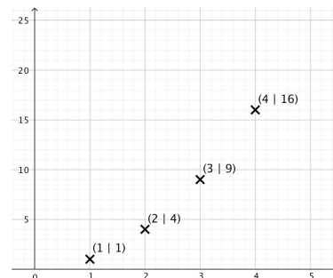
Abb. 4.17: Graph einer Folge
