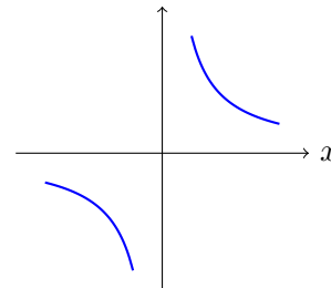
Abb. 5.18: f(x) = \frac{1}{x}
