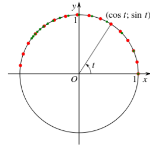
Abb. 3.13: Der Kreis
