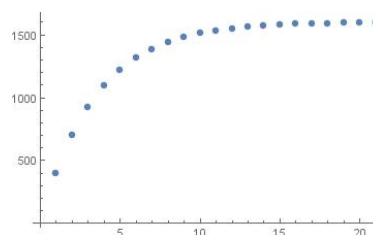
Abb. 4.9: Graph der Folge (m_n)
