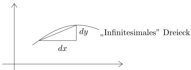
Abb. 5.26: Tangentensteigung mittels „unendlich kleiner“ Dreiecke.
