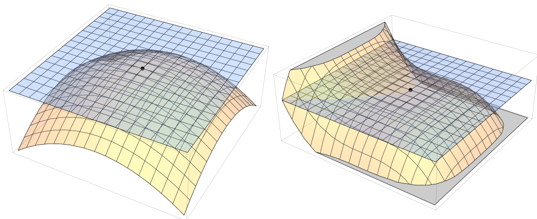
Abb. 5.24: Die Tangentialebene als lineare Bestapproximation an den Graphen von Funktionen f : \mathbb{R}^2 \rightarrow \mathbb{R} lokal um den eingezeichneten Punkt
