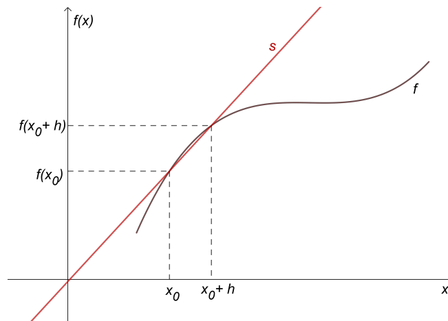
Abb. 5.15: Geraden zwischen den Punkten (x_0, f(x_0)) und (x_0 + h, f(x_0 + h))
