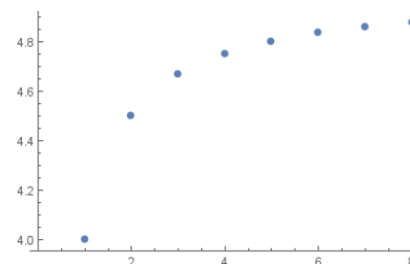
Abb. 4.6: Graph einer reellen Folge (a_n) .
