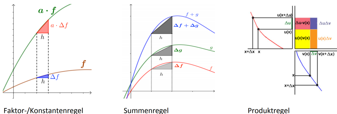
Abb. 5.38: Geometrische Interpretationen von Ableitungsregeln
