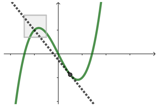
Abb. 5.5: Tangente als Schmiegegerade aber nicht als Stützgerade
