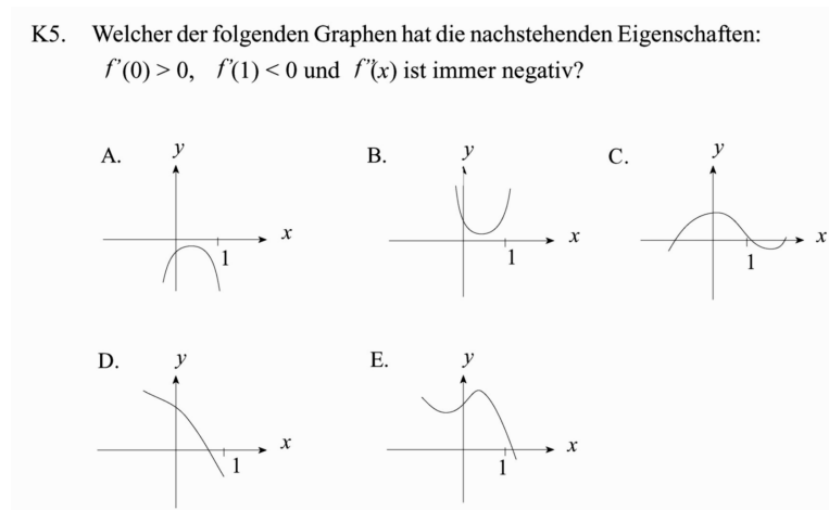
Abb. 5.39: Aufgabe aus TIMSS III zur Deutung formaler Bedingungen an Funktionsgraphen.
