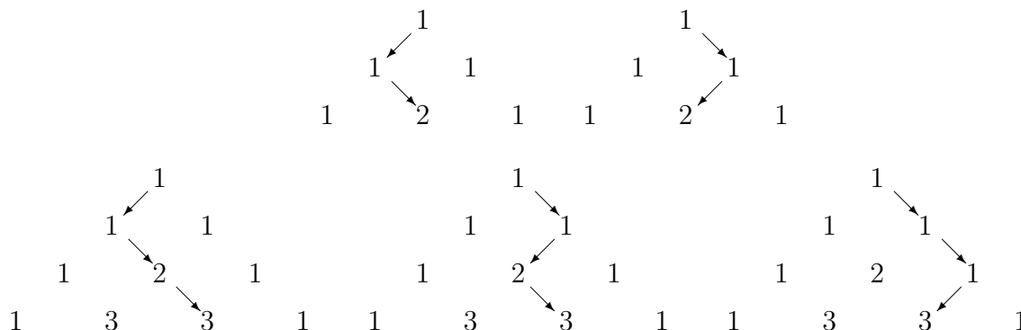
ABBILDUNG 2.1. Pascalsches Dreieck
