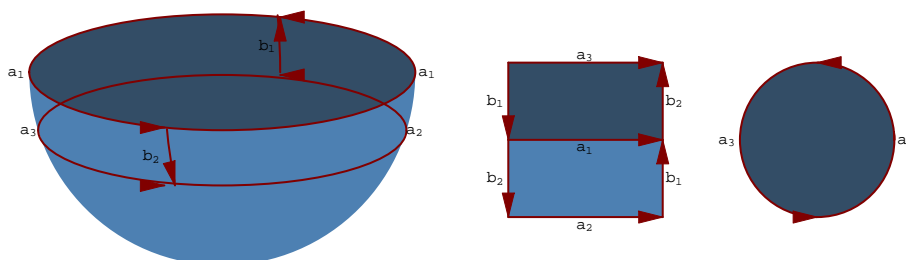
Kreuzhaube
