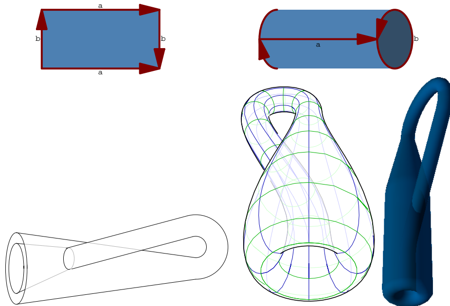
Klein'sche Flasche
