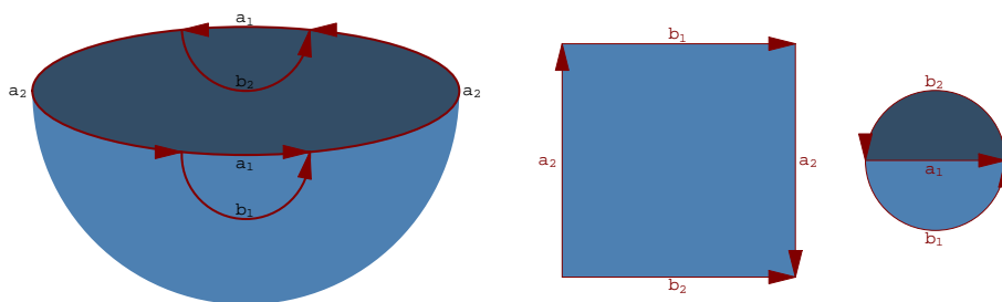
Projektive Ebene
