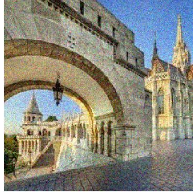
(d) Choice (II): M_2^k = \sigma_k^{-1} \text{Id}
