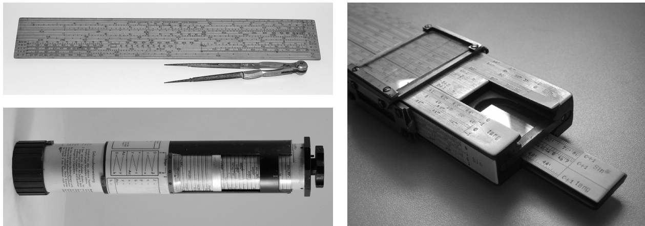
Abbildung 11: links: Gunterscale mit Zirkel, Dennert & Pape Höhenrechenschieber MHR1, rechts: der große Nelting, Dennert & Pape Nr. 29
