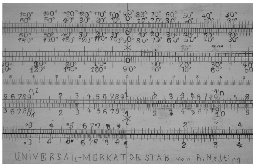
Abbildung 10: Händisch erstellte Skalen auf Neltings Prototyp für einen Mercatorrechenstab
