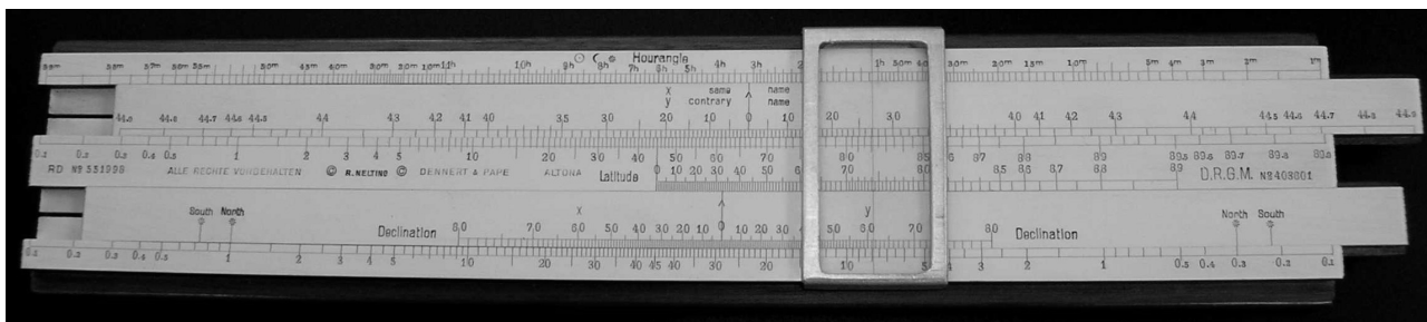
Abbildung 5: Nr. 28 – Azimutstab (englische Version)
