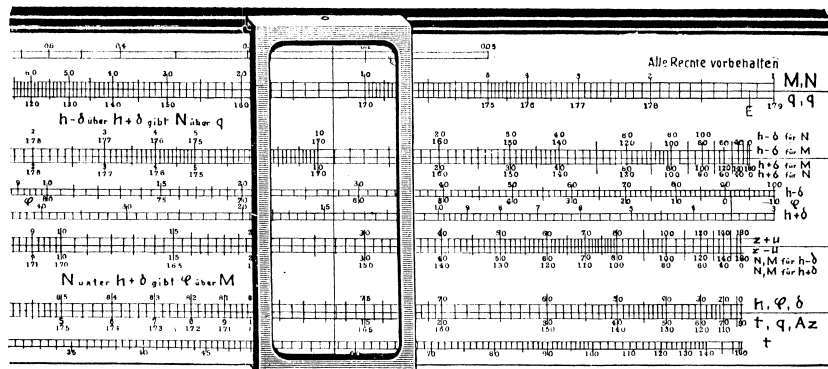
Abbildung 9: Skalenbild Nr. 31 (Katalog 1919 [3])
