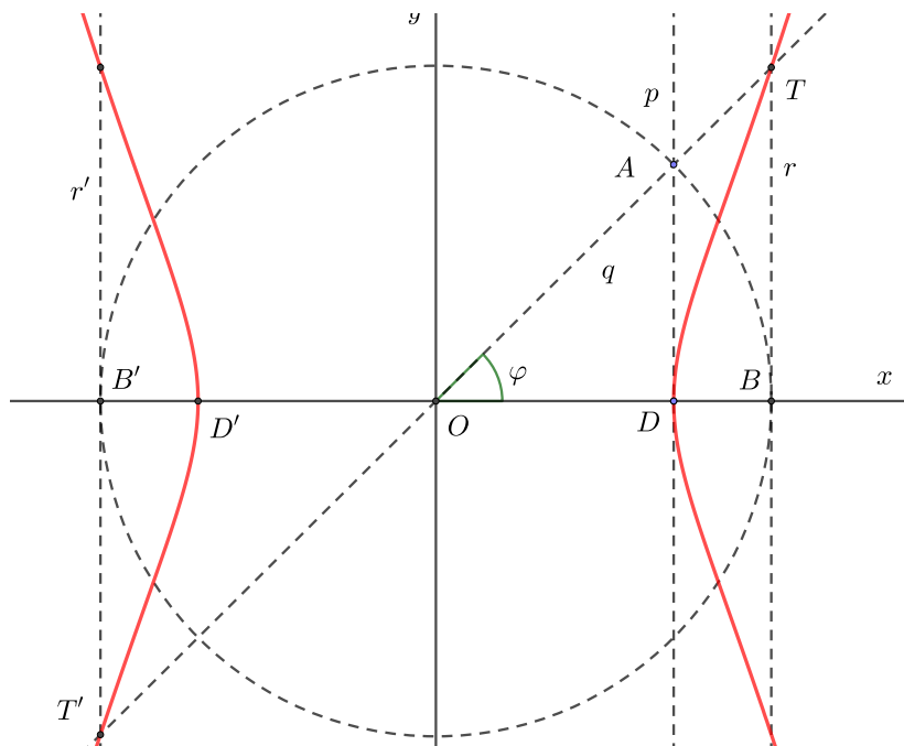
Abbildung 1: Konstruktion eines Punktes der Kampyle.
