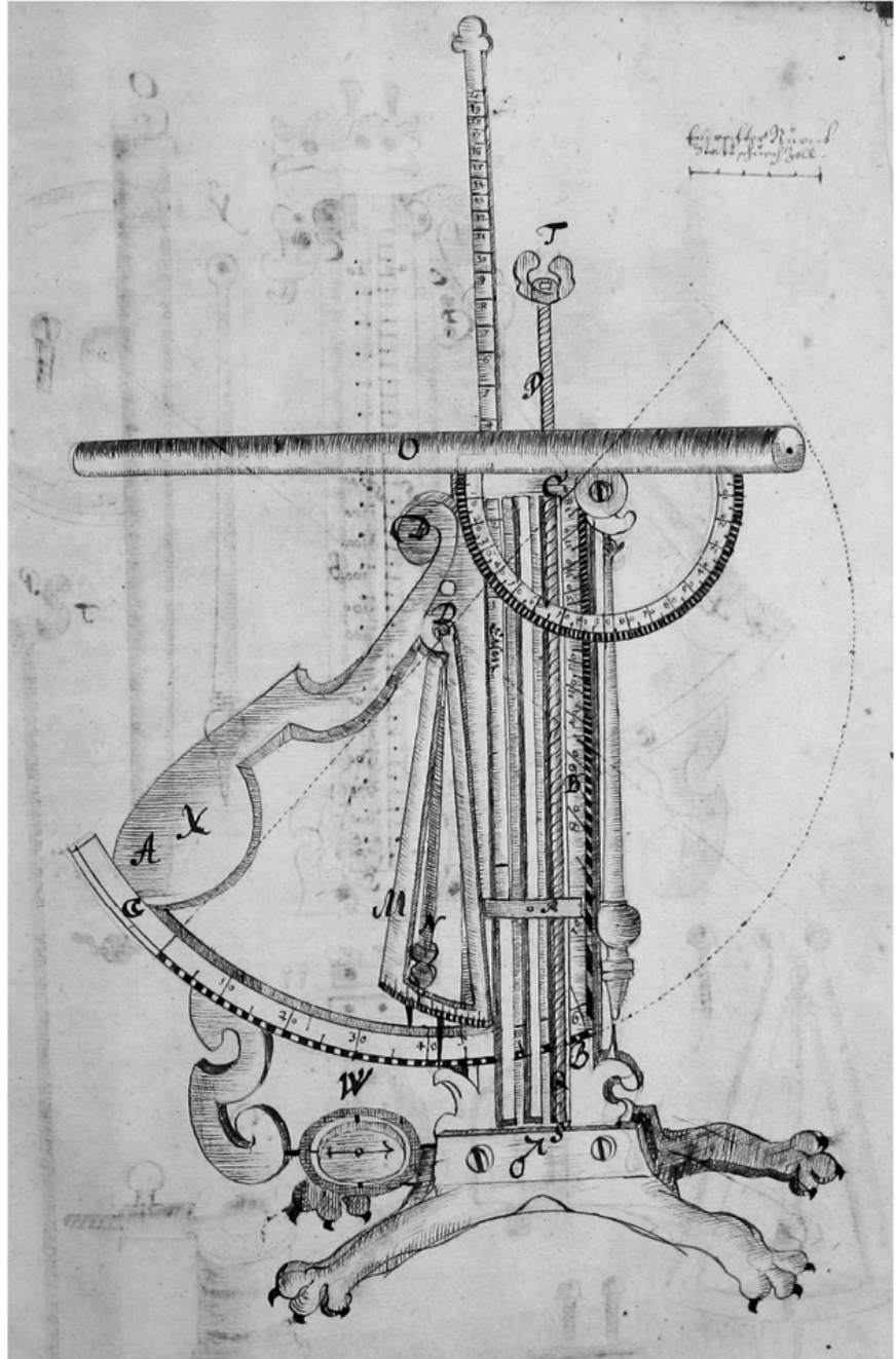
Geschützaufsatz in J. C. Kaukol, Püchsenmeisterey-Buch 1669, fol. 28 r
