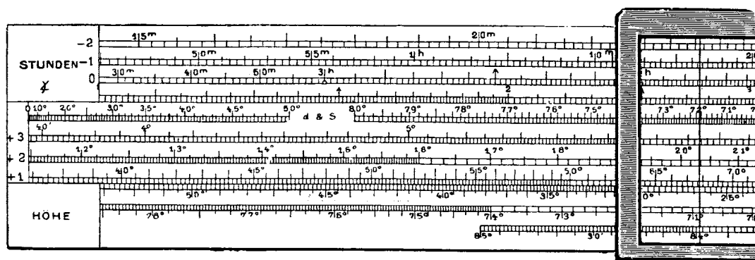
Abbildung 8: Nr. 30 – Skalenbild Gestirn-Höhen-Azimutstab – aus Katalog 1924 [3]
