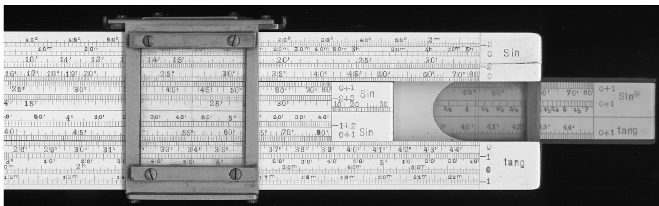
Abbildung 7: Nr. 29 – der große Nelting, Grad und Zeit-Skalen für sin und tan
