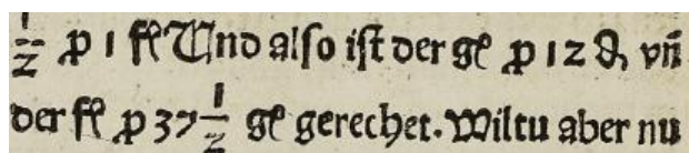
Abb. 2: Widmanns Lösung (84 v )
