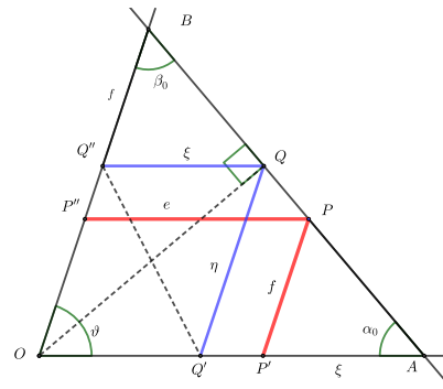
Abb. 3: Philonsche Gerade durch den Punkt P und seinen zugeteilten Punkt Q .
