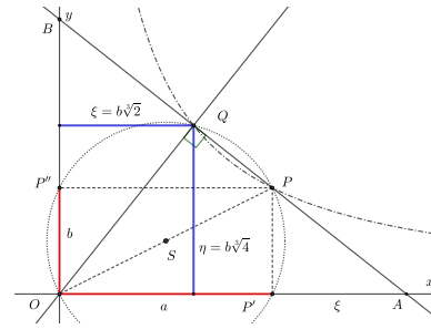
Abb. 7: Würfelverdoppelung.
