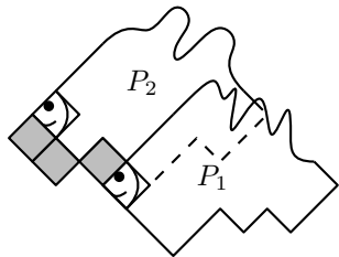
C_2^\bullet(P_1, P_2, i)
